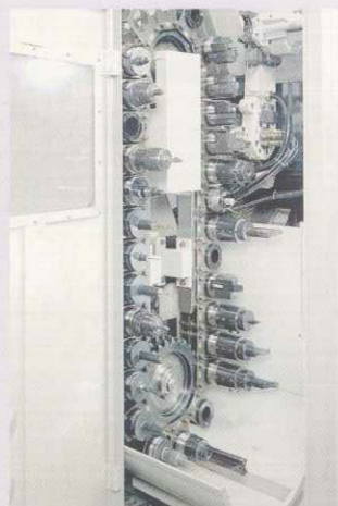
30本ツールマガジン(INTEGREX 50&70)
