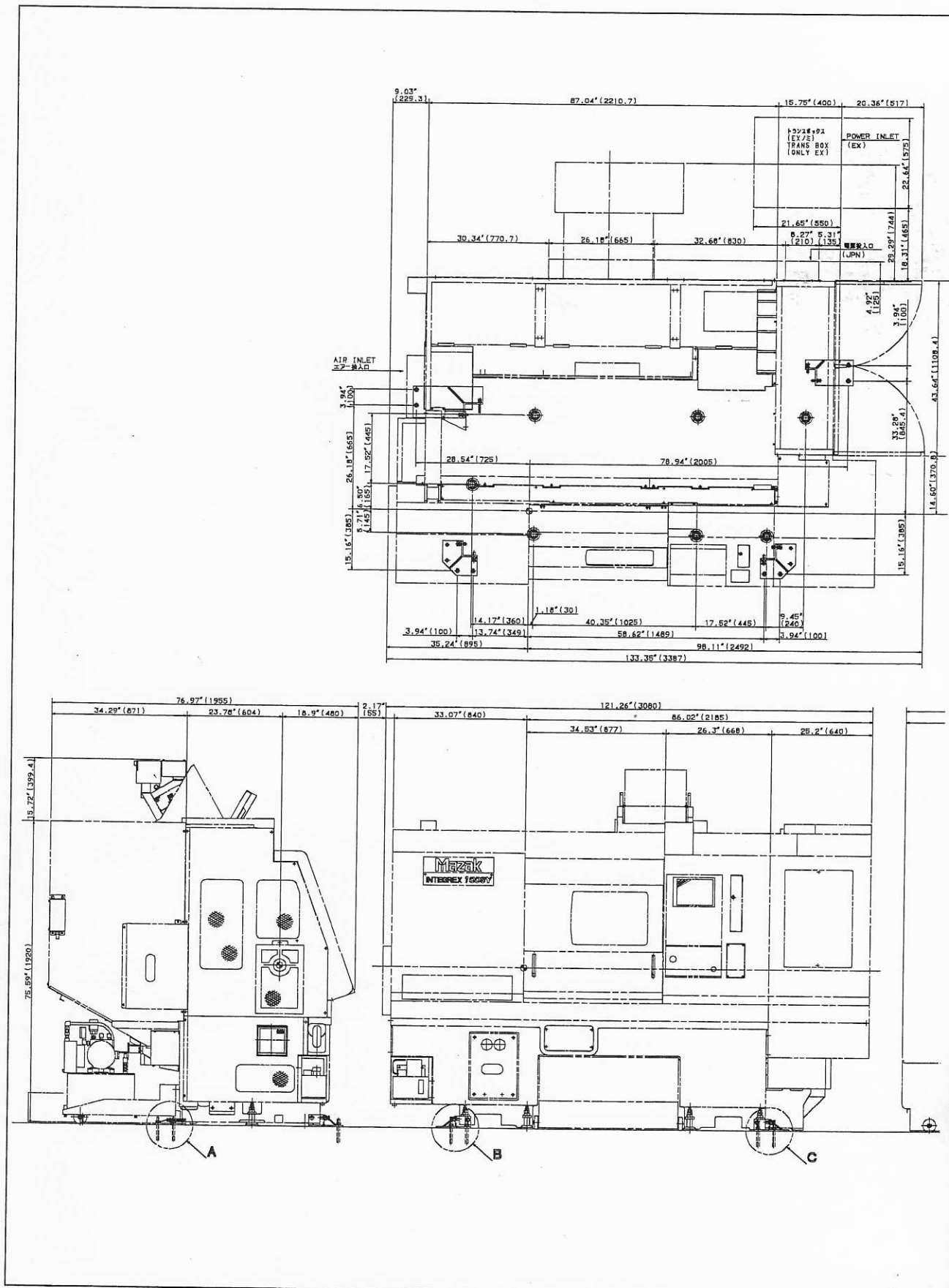
Fig. 3-7 ドライブット方式本機固定位置図 INTEGREG 100-IISY (ワーク搬出コンベア無)
